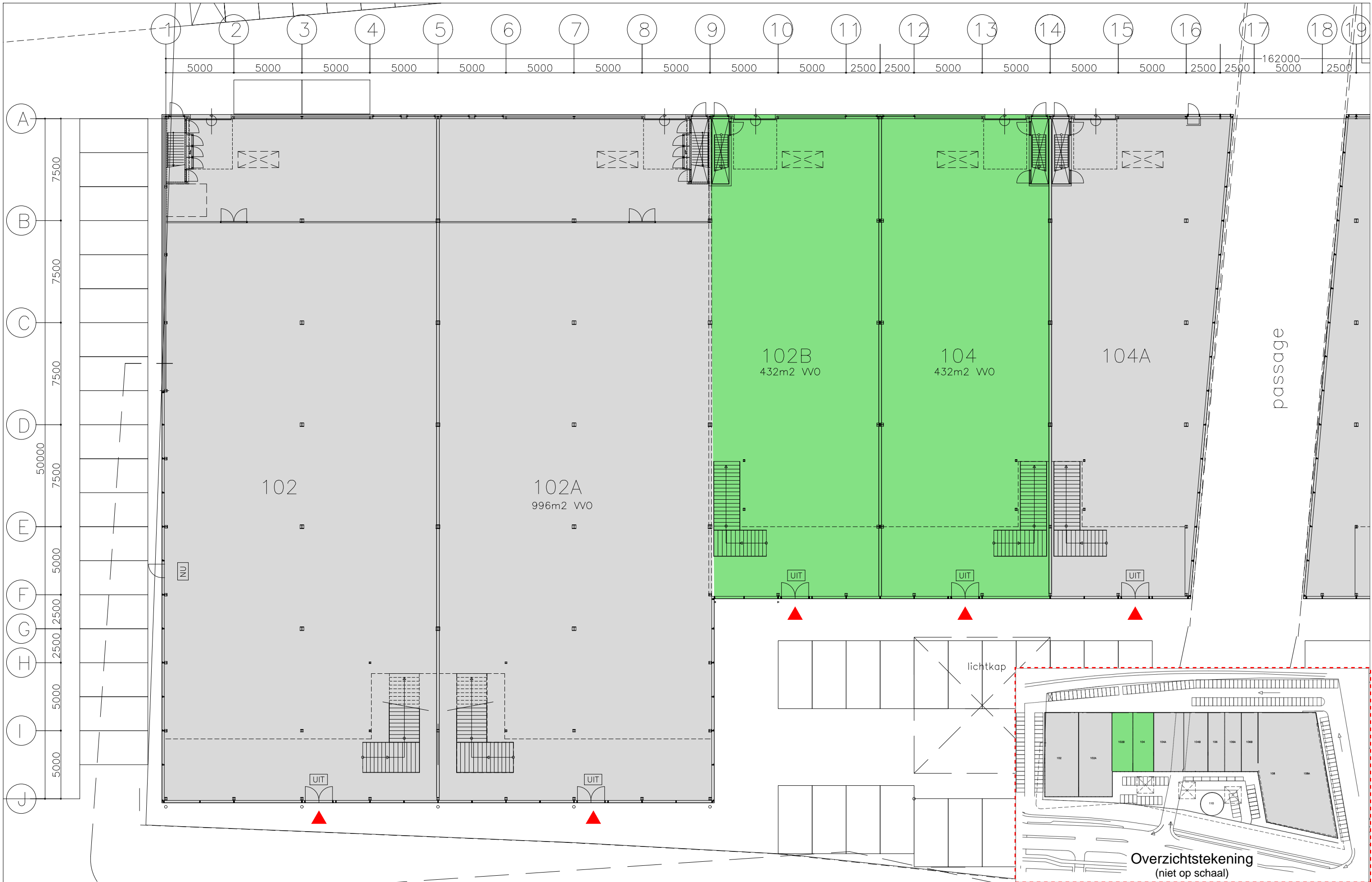
Verhuurtekening Begane Grond Parallelweg 102B t/m 104, Beverwijk (Woonplaza)
